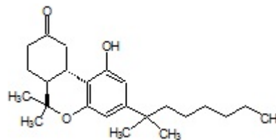
Nabilone
